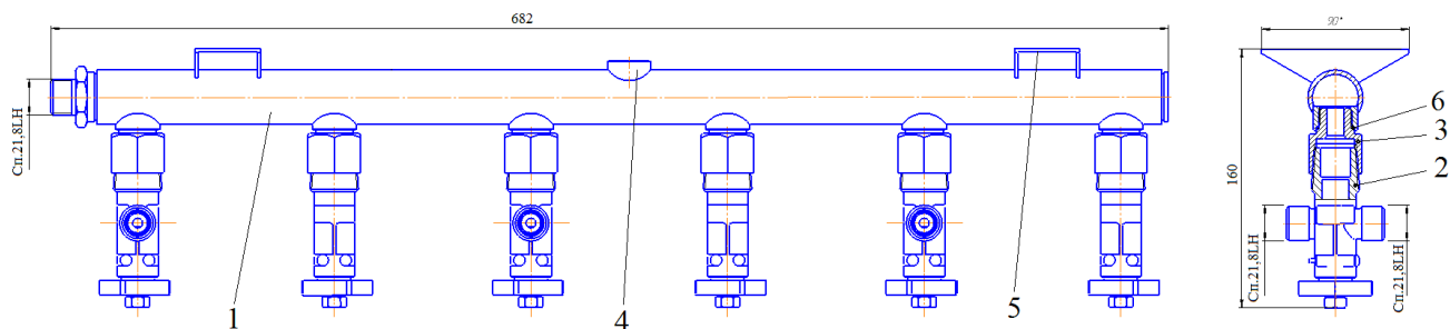
Рис.1 Коллектор газовый КР-03 ДЖЕТ 245 00 00 00-36
